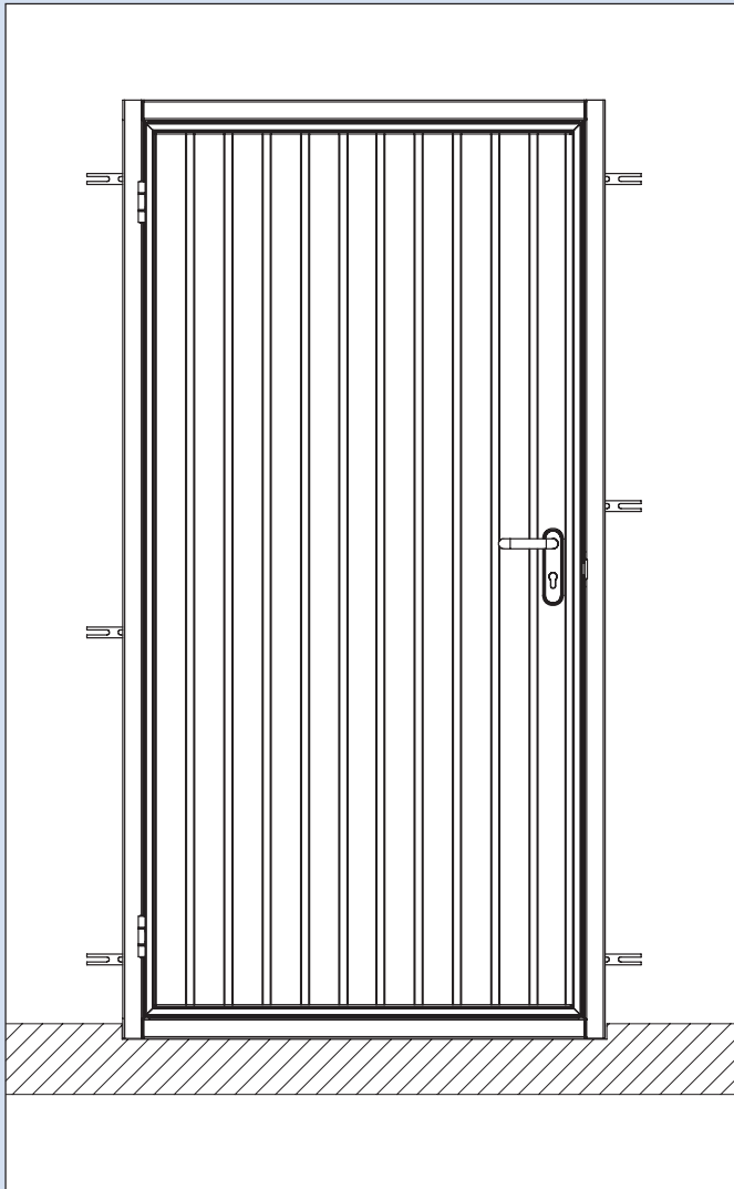
Frontansicht mit Ankeranordnung
