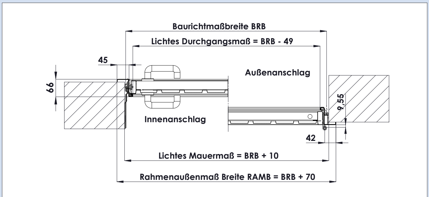
Horizontalanschnitt am Beispiel Innenanschlag
